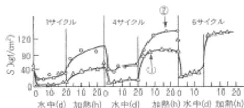
図3-26 塗膜の浸水-加熱サイクル老化による内部応力の変化 1)
