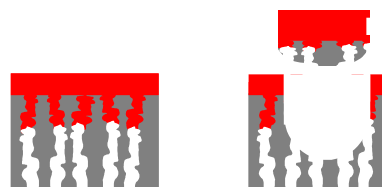
根付き塗膜 JIS 5.7 7 材法での破壊状況
